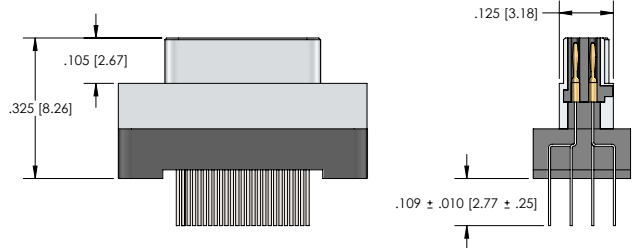
PLUG (PINS)
