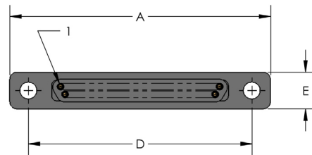
PLUG (PINS)
