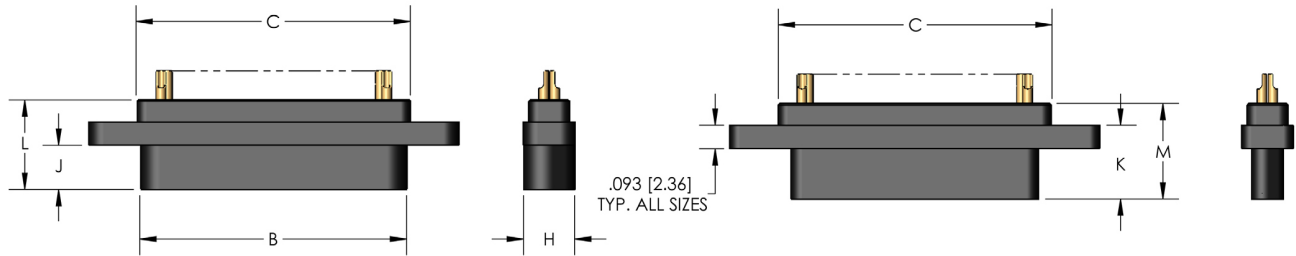
RECEPTACLE (SOCKETS)
