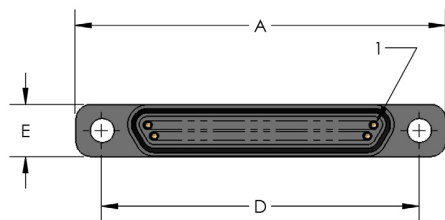
RECEPTACLE (SOCKETS)
