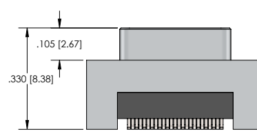
PLUG (PINS)
