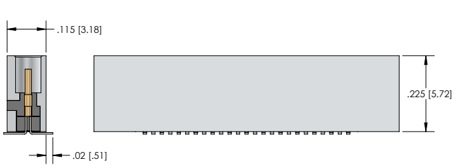
RECEPTACLE (SOCKETS)
